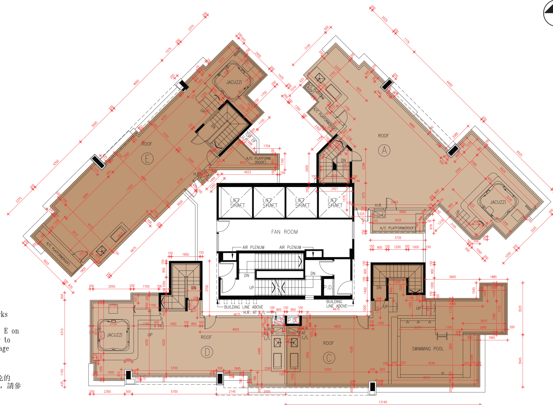
Tower 5 Roof Plan 第5座 天台樓面平面圖
